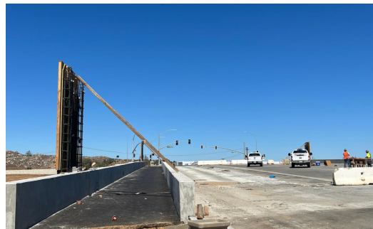
Progreso en el camino ecuestre sobre el puente Placentia Ave. en la I-215
