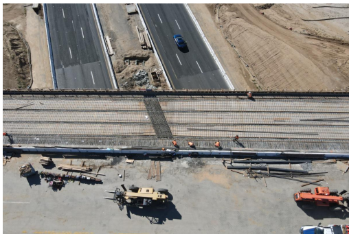
Cuadrillas preparan para verter concreto en el puente de Placentia Ave. sobre la I-215 hacia.
